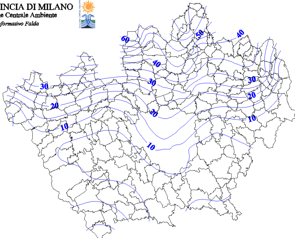
CARTA DELLA SOGGIACENZA DELLA FALDA FREATICA NELLA PROVINCIA DI MILANO (metri dal p.c.) MARZO 2002
